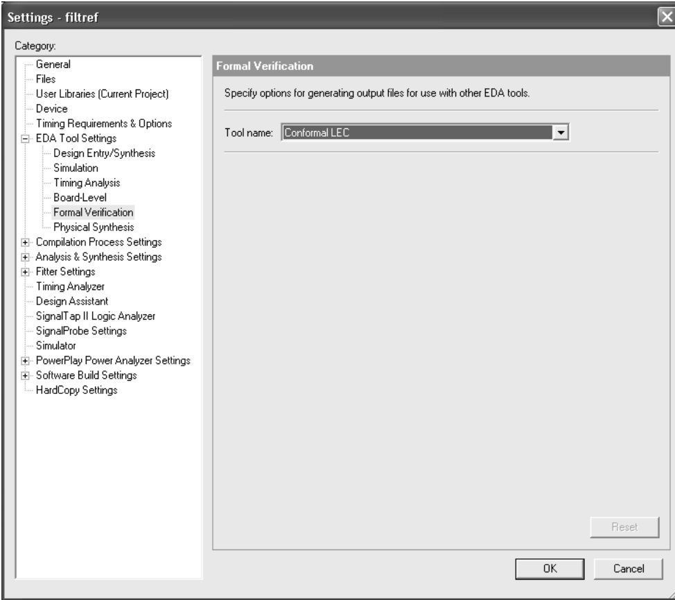
图 3. Settings 对话框的 Formal Verification 页面
