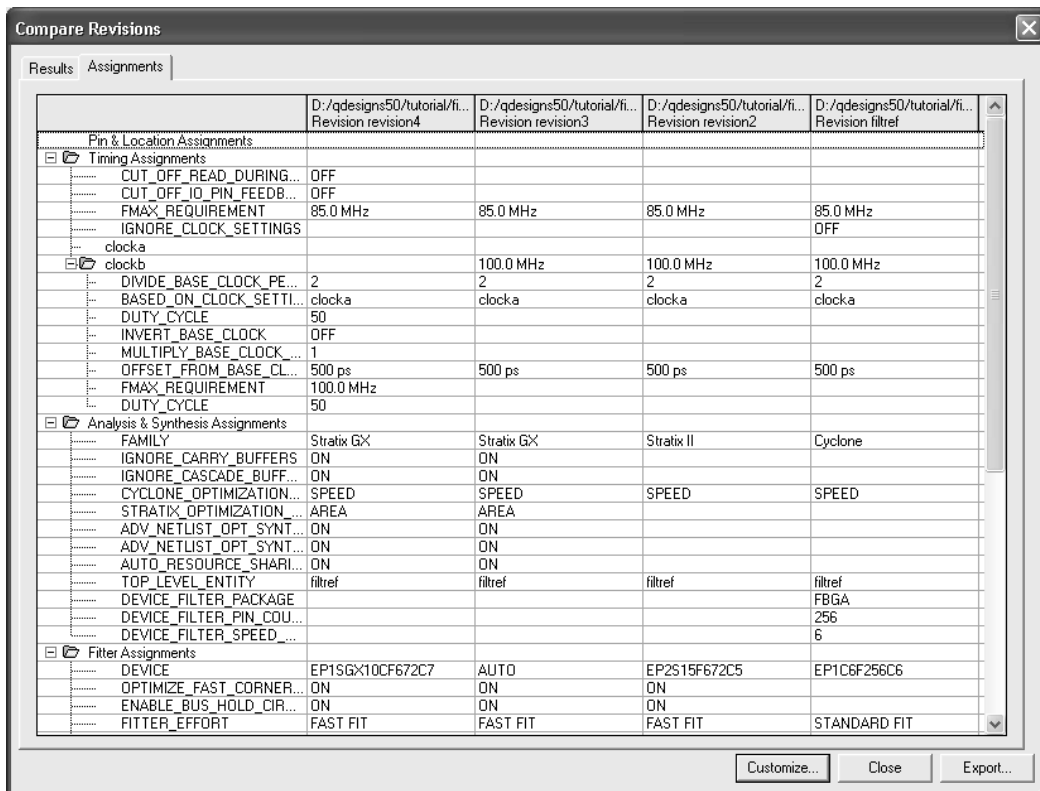
图 5. Compare Revisions 对话框的 Assignments 标签选项
