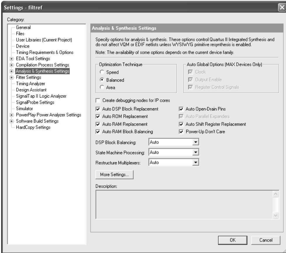
图 4. Settings 对话框的 Analysis & Synthesis 设置页面
