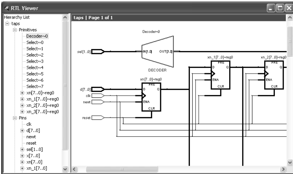
图 6. RTL Viewer 窗口
