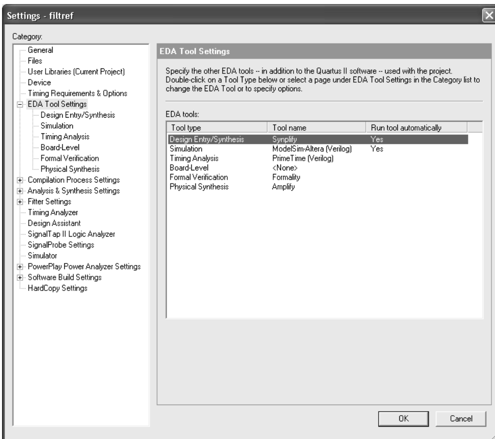
图 8. Settings 对话框的 EDA Tool Settings 页面
