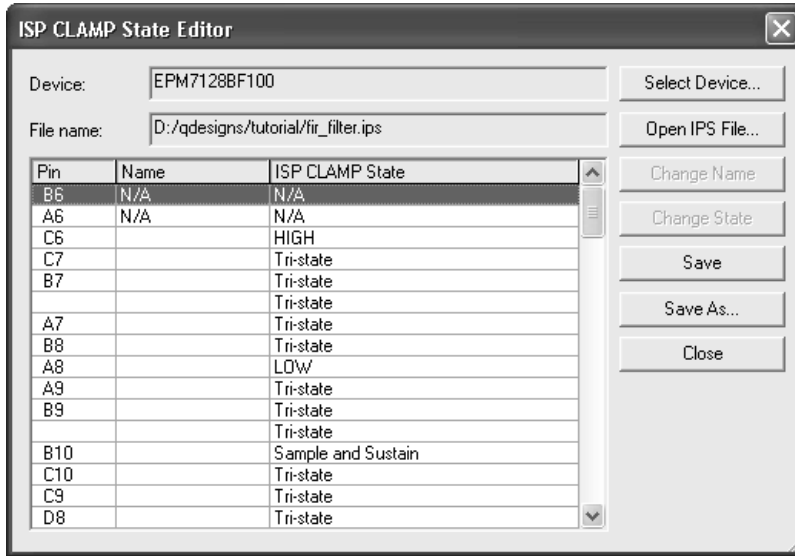
图 4. ISP CLAMP State Editor 对话框
