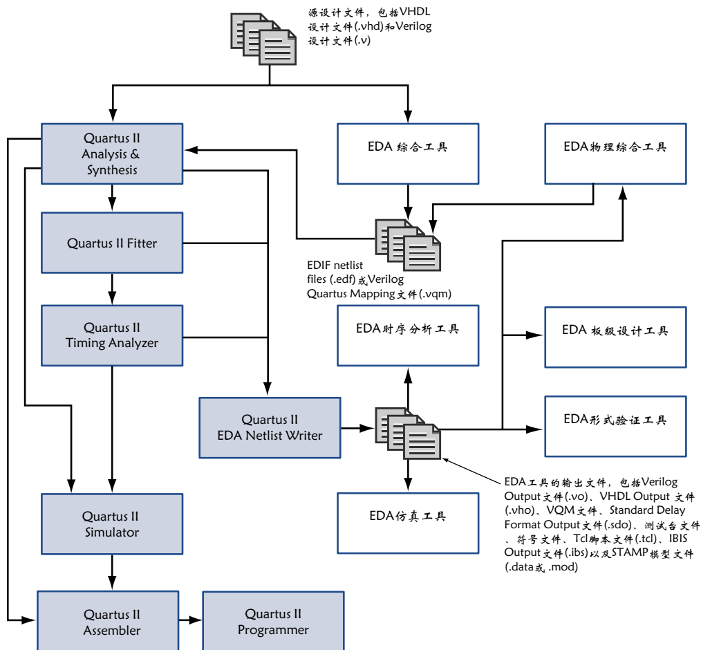
图 7. EDA 工具设计流程
