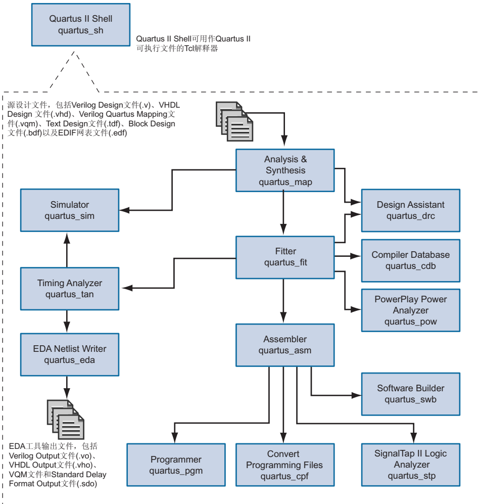
图 9. 命令行设计流程
