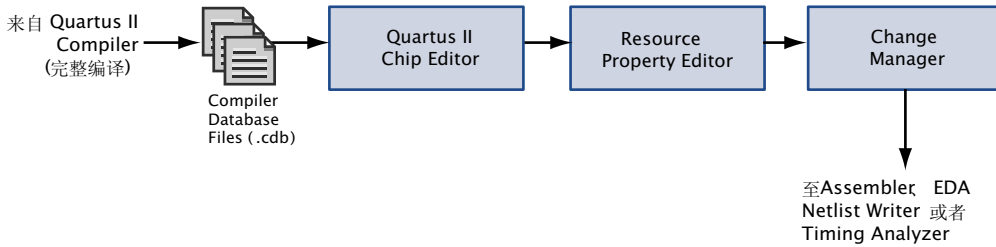
图 1. 工程更改管理设计流程
