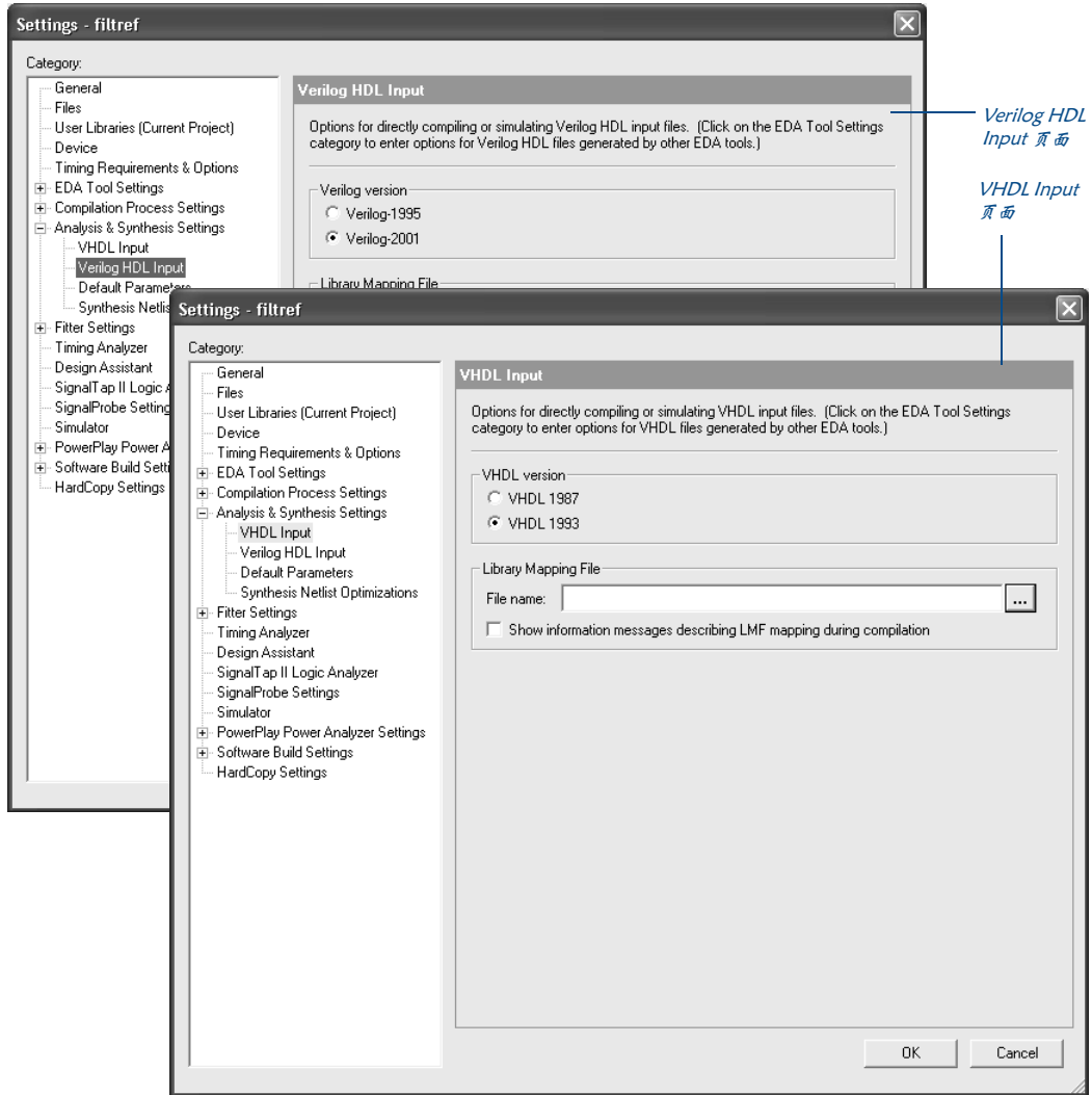
图 2. Settings 对话框的 Verilog HDL 和 VHDL Input 页面
