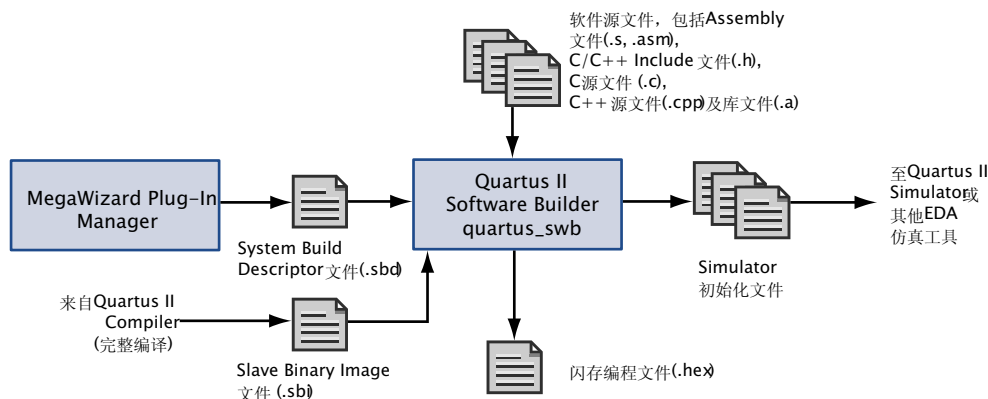
图 1. 闪存编程文件流程
