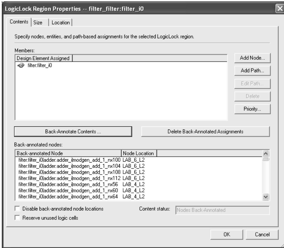
图 3. LogicLock Region Properties 对话框
