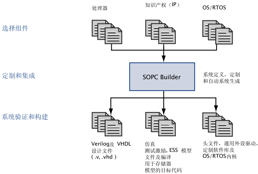
图 1. SOPC Builder 设计流程
