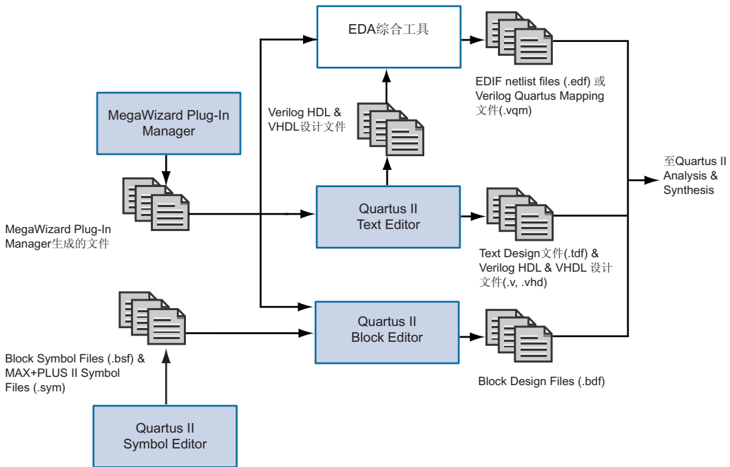
图 1. 设计输入流程
