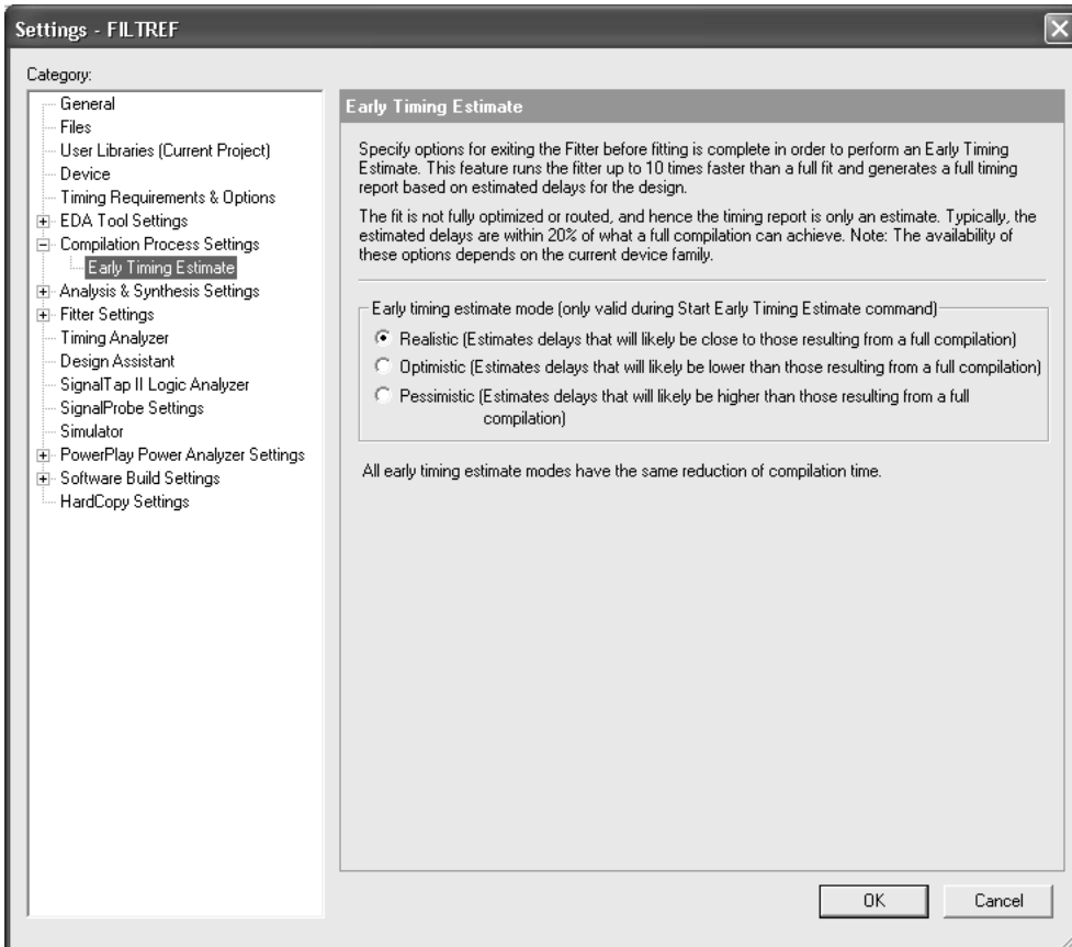
图 4. Settings 对话框的 Early Timing Estimate 页面
