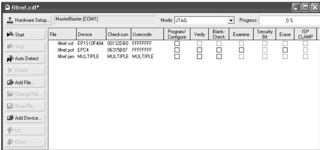
图 2. Programmer 窗口
