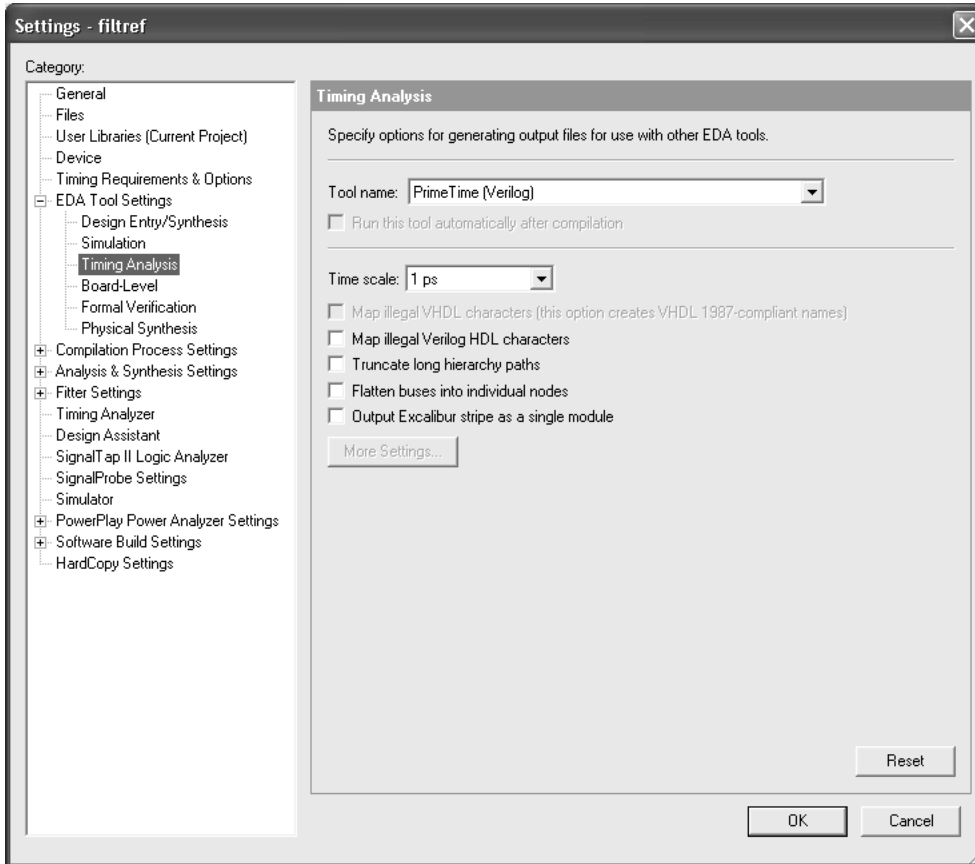
图 9. Settings 对话框的 EDA Tool Timing Analysis 页面
