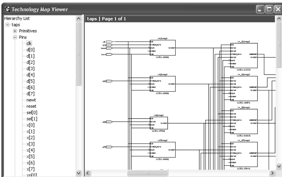
图 9. Technology Map Viewer 窗口
