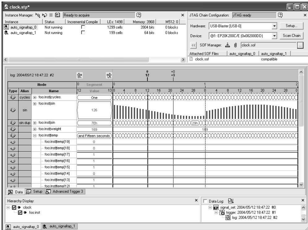
图 5. SignalTap II 波形视图
