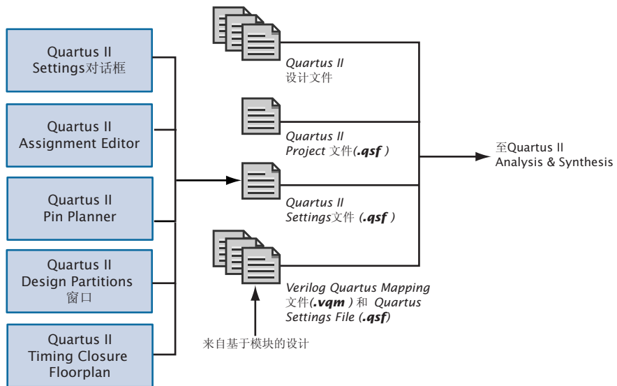
图 1. 约束和分配输入流程
