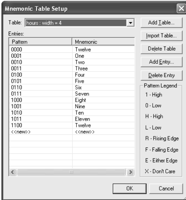
图 6. Mnemonic Table Setup 对话框
