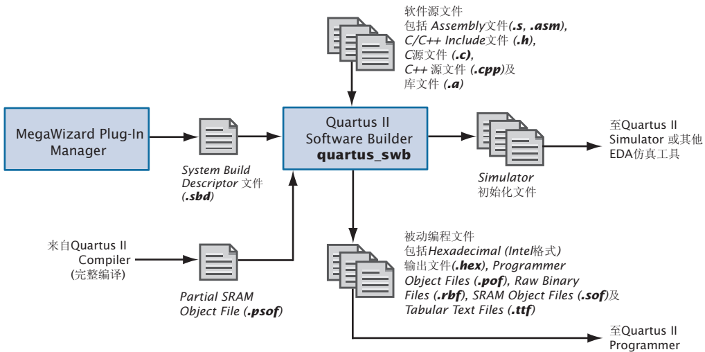
图 2. 被动编程文件流程
