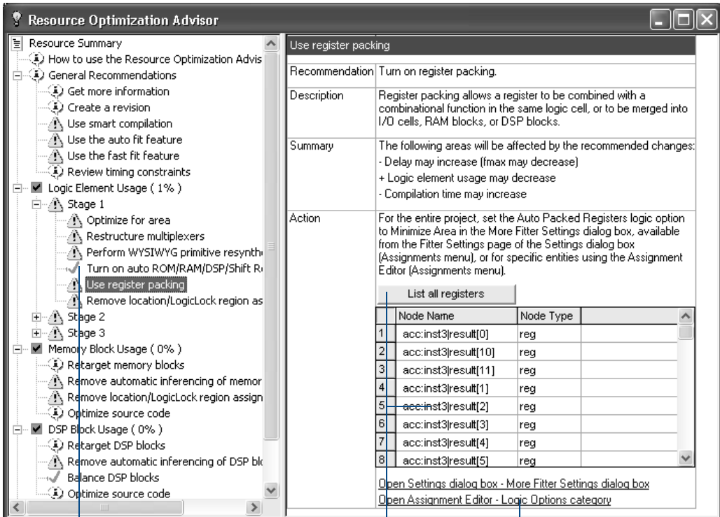
图 7. Resource Optimization Advisor 建议页面
