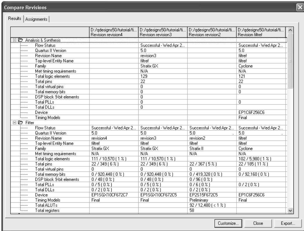
图 4. Compare Revisions 对话框的 Results 标签选项
