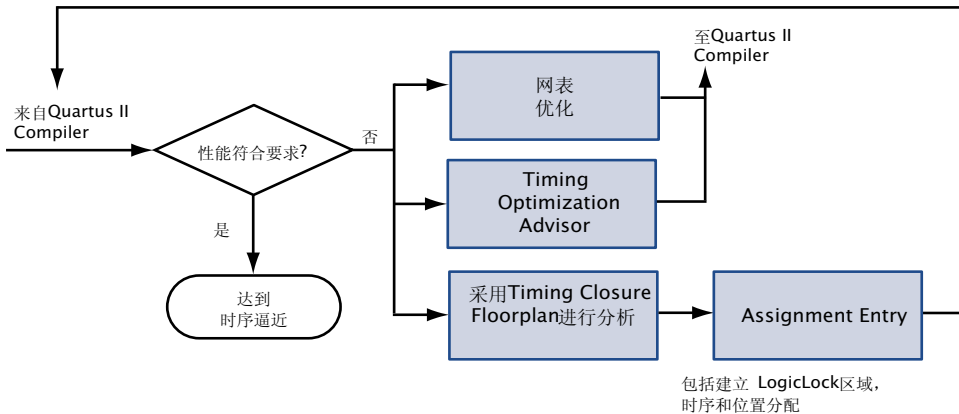
图 1. 时序逼近流程
