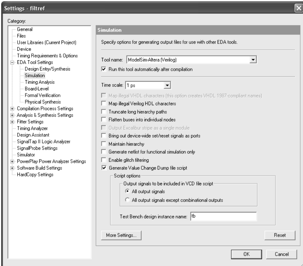
图 2. Settings 对话框的 EDA Tool Simulation 页面
