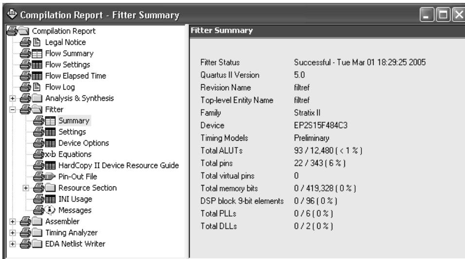
图 4. Report 窗口的 Fitter 部分
