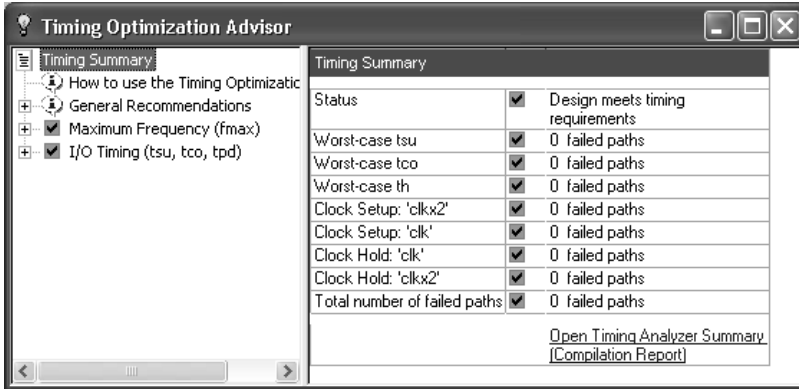
图 3. Timing Optimization Advisor 初始页面
