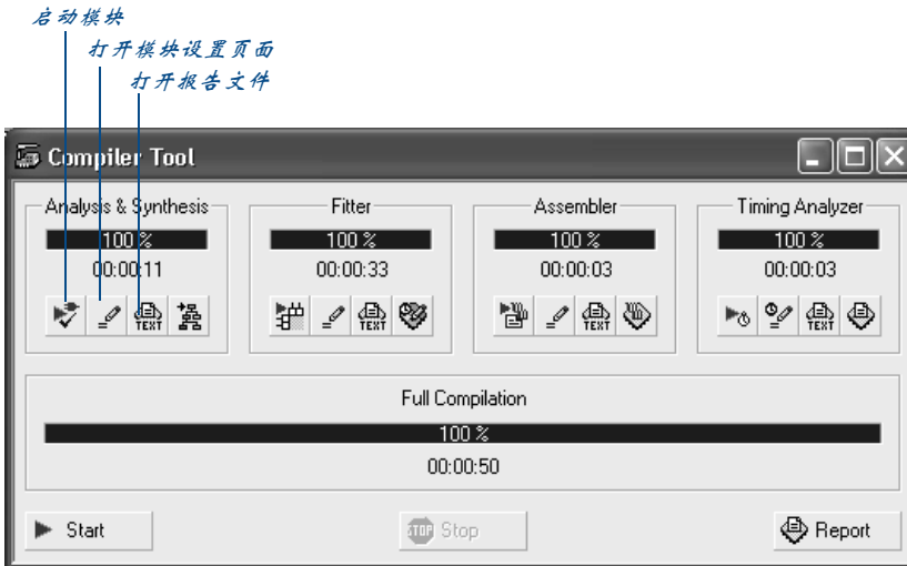
图 4. Compiler Tool 窗口
