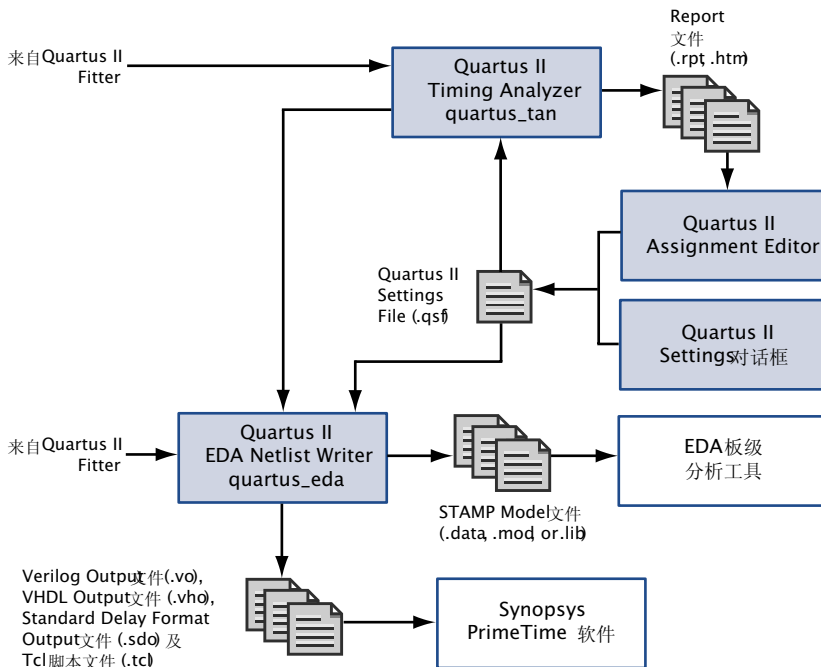
图 1. 时序分析流程
