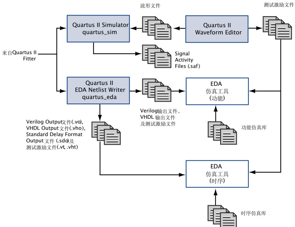
图 1. 仿真流程
