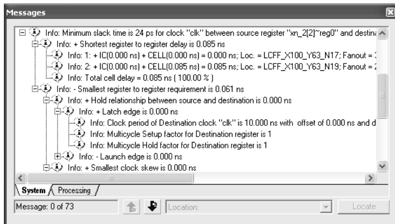
图 6. List Paths 命令的输出
