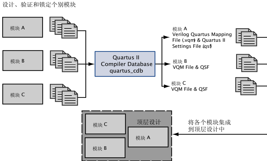
图 1. 基于模块的设计流程
