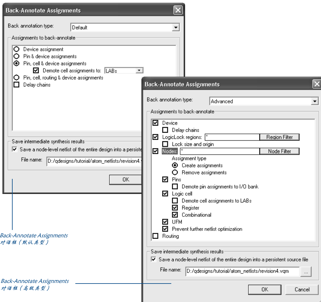
图 11. Back-Annotate Assignments 对话框
