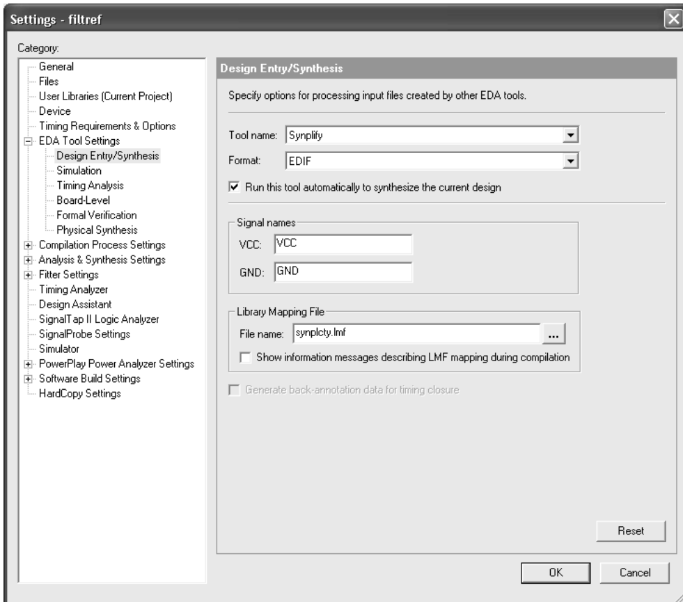
图 3. Settings 对话框的 EDA Tool Design Entry & Synthesis 页面
