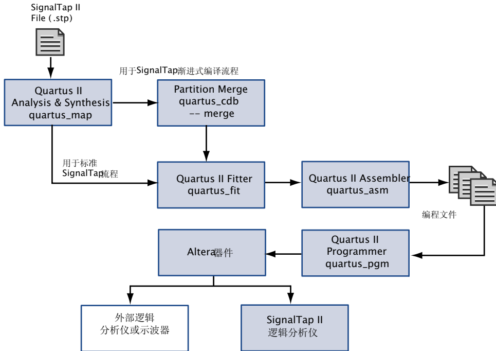
图 1. SignalTap II 调试流程
