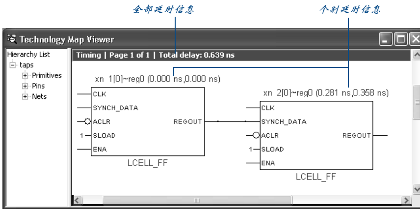
图 8. Technology Map Viewer 窗口——延时信息
