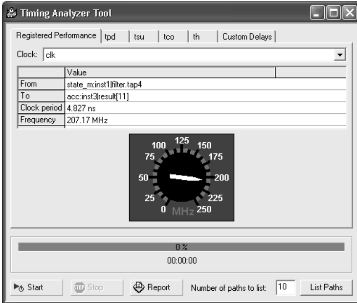
图 3. Timing Analyzer Tool
