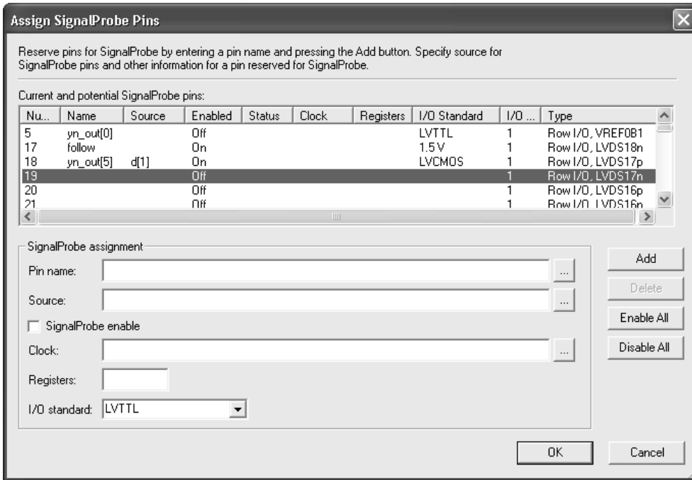
图 7. Assign SignalProbe Pins 对话框
