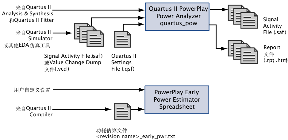
图 1. PowerPlay Power Analysis 流程
