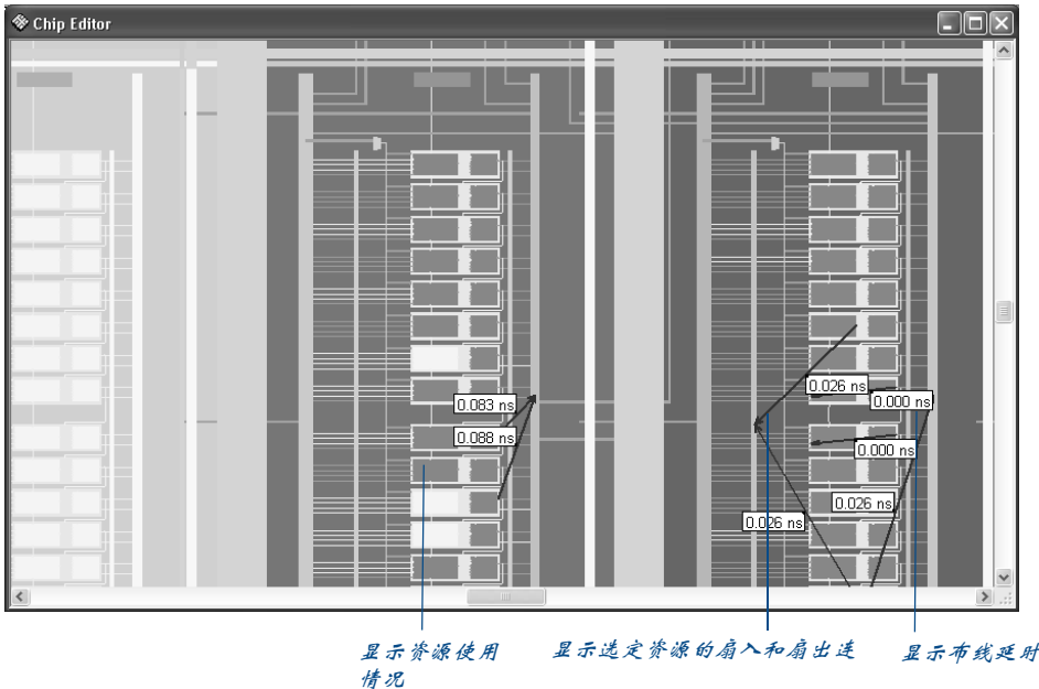
图 2. Chip Editor
