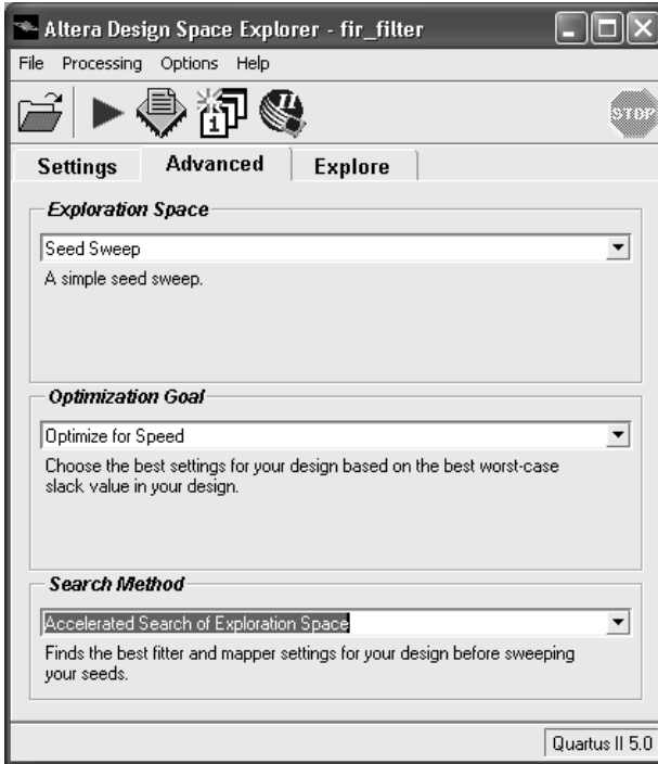
图 9. Design Space Explorer 的 Advanced 标签选项
