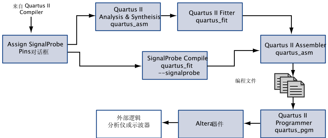
图 2. SignalProbe 调试流程
