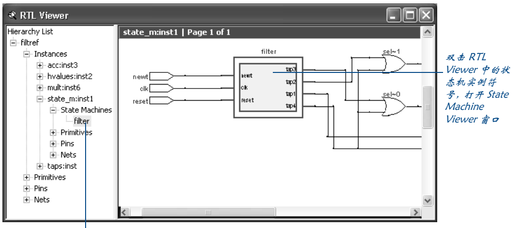
图 7. RTL Viewer 窗口中的状态机实例
