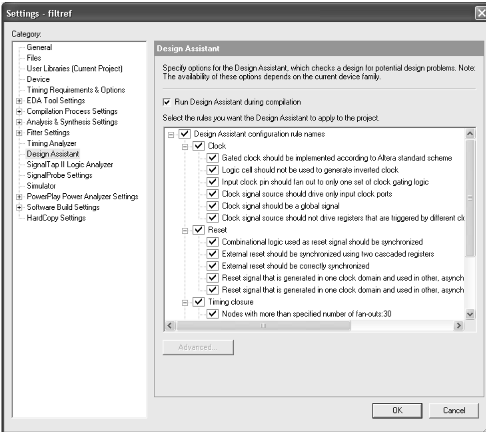
图 5. Settings 对话框的 Design Assistant 页面
