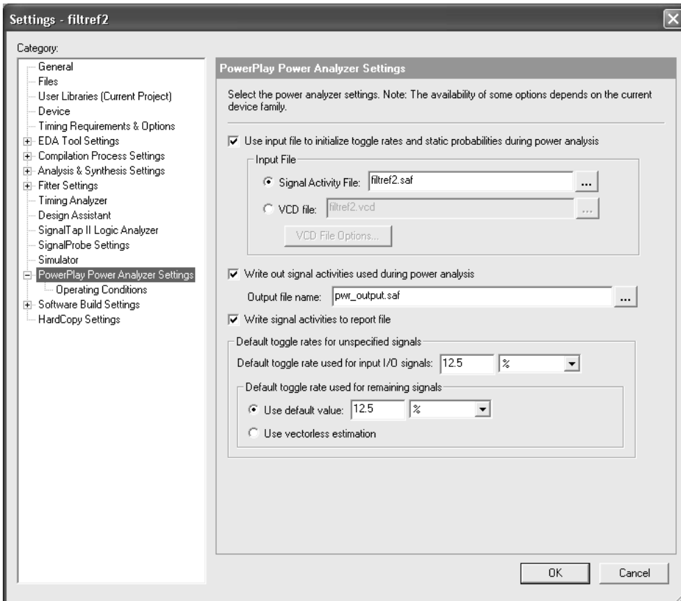
图 3. PowerPlay Power Analyzer Settings 页面
