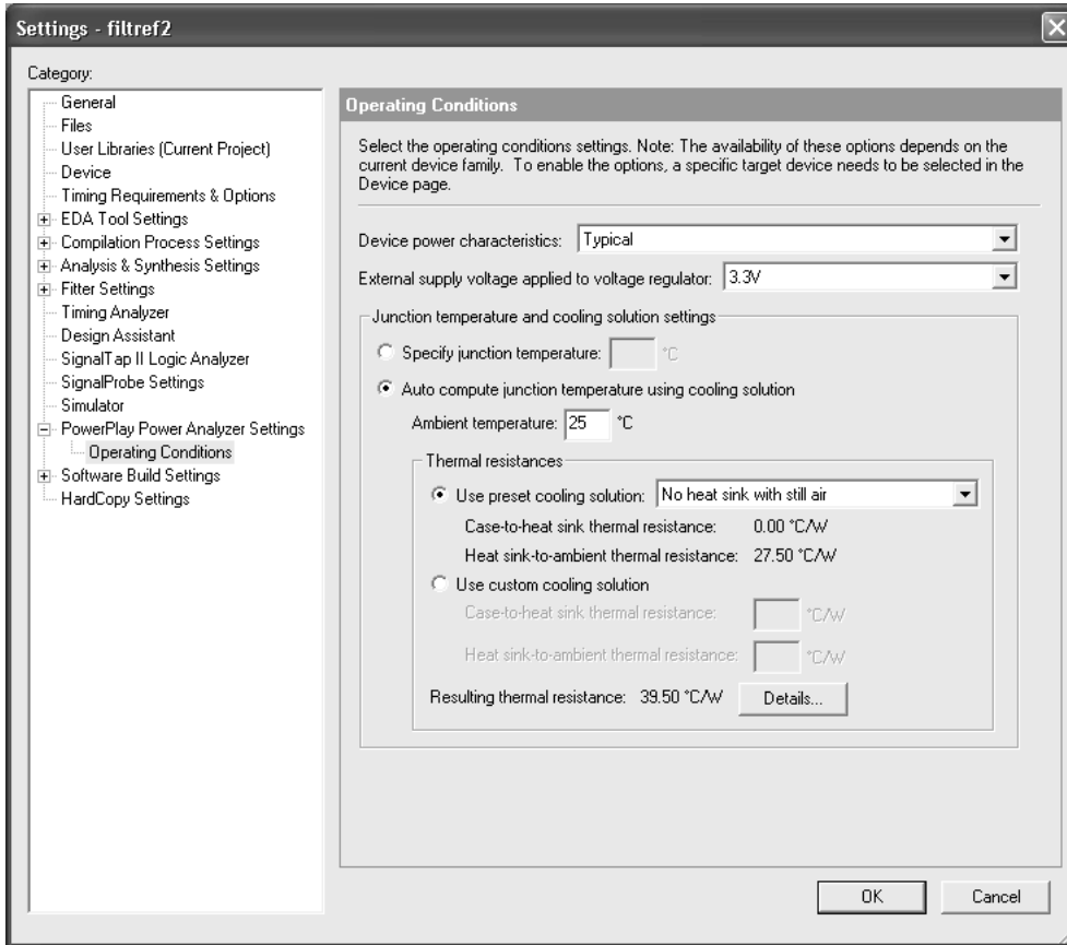
图 4. Operating Conditions 页面
