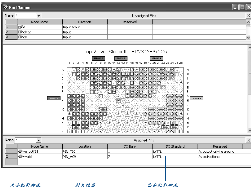
图 3. Pin Planner
