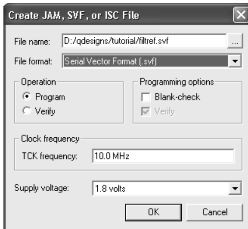
图 3. Create JAM, SVF, or ISC File 对话框
