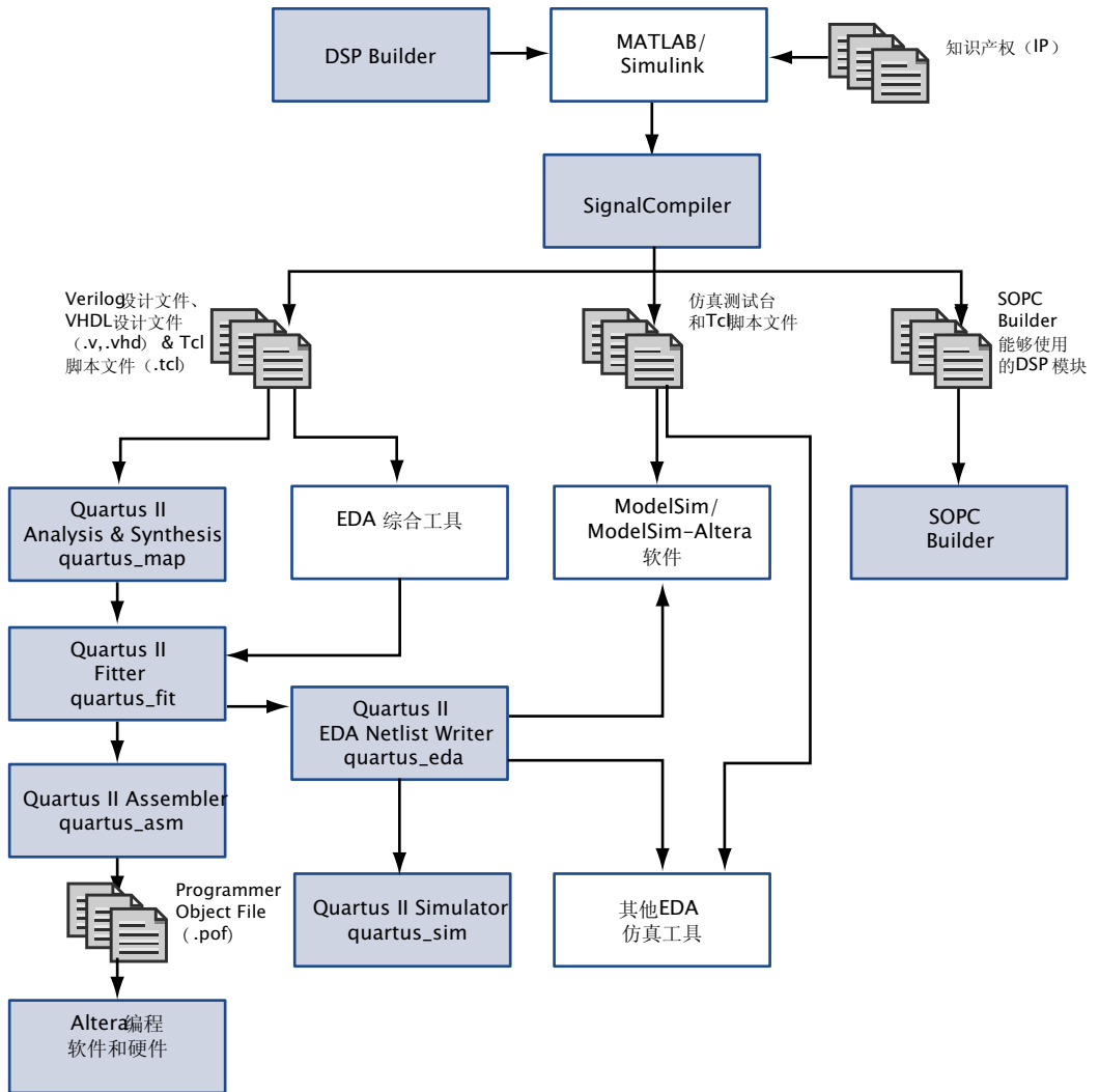
图 2. DSP Builder 设计流程
