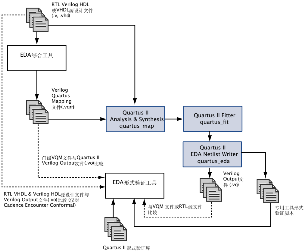
图 1. 形式验证流程
