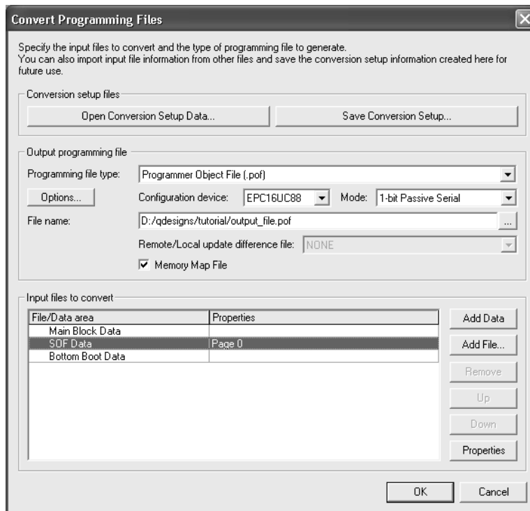
图 5. Convert Programming Files 对话框
