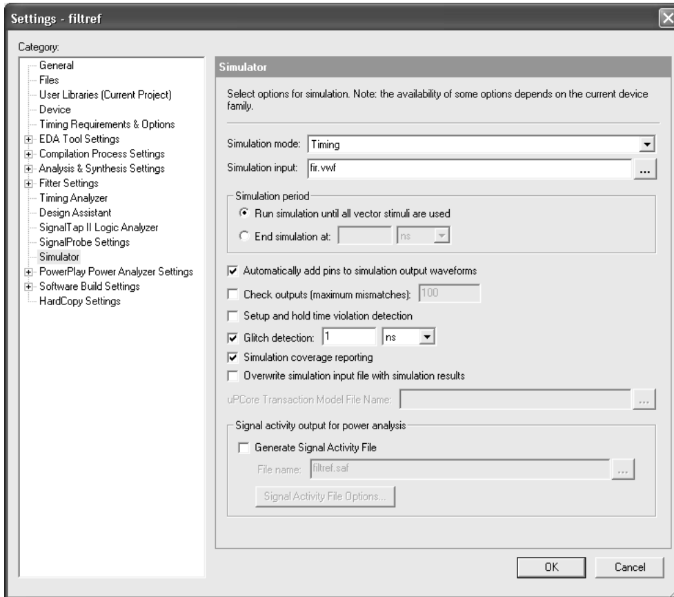
图 3. Settings 对话框的 Simulator 页面
