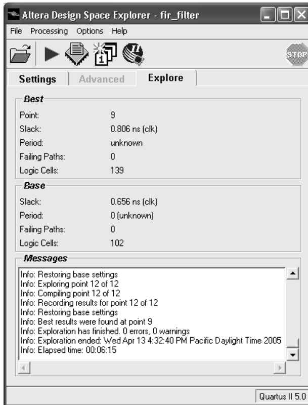
图 10. Design Space Explorer 的 Explore 选项标签
