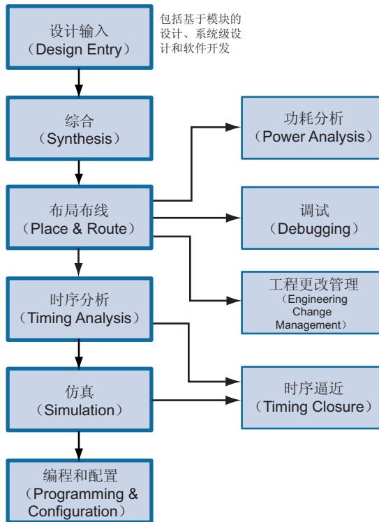
图 1. Quartus II 设计流程
